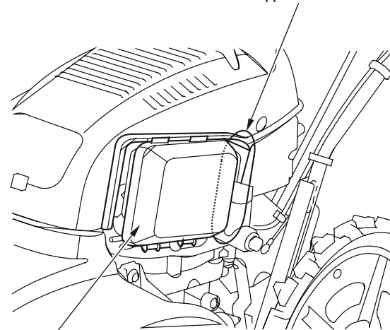
ЗАМОК ВОЗДУШНОГО ФИЛЬТРА
