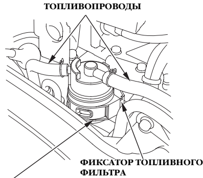
ТОПЛИВОПРОВОДЫ ФИКСАТОР ТОПЛИВНОГО ФИЛЬТРА ЛЕНТОЧНЫЙ ХОМУТ
