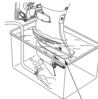
АНТИКАВАТАЦИОННАЯ ПЛИТА
