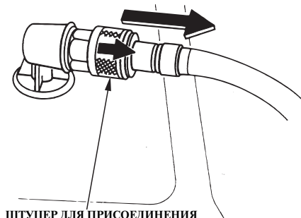
ШТУЦЕР ДЛЯ ПРИСОЕДИНЕНИЯ ТОПЛИВОПРОВОДА
