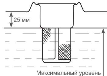
Рис.8 Максимальный уровень топлива
