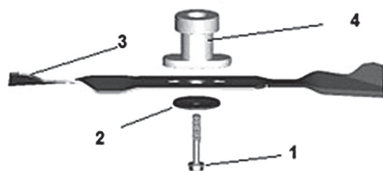
Рис. 18 Обслуживание ножа
