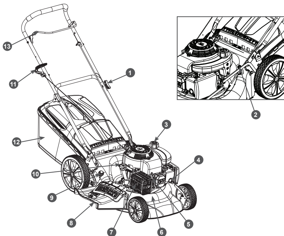
Рис. 1 Основные узлы и органы управления газонокосилки LM4622
