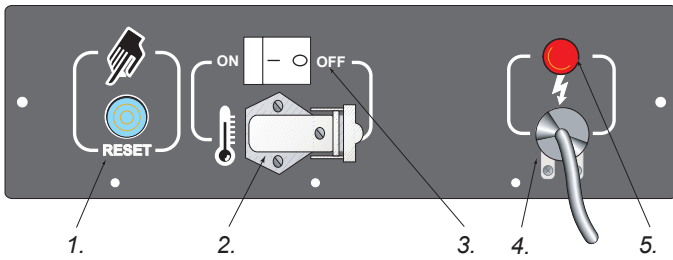
Slika 6 – Električna ploča.
