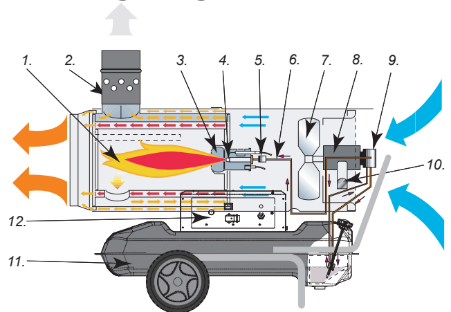
Abbildung 4 - Betriebsschema BV.
