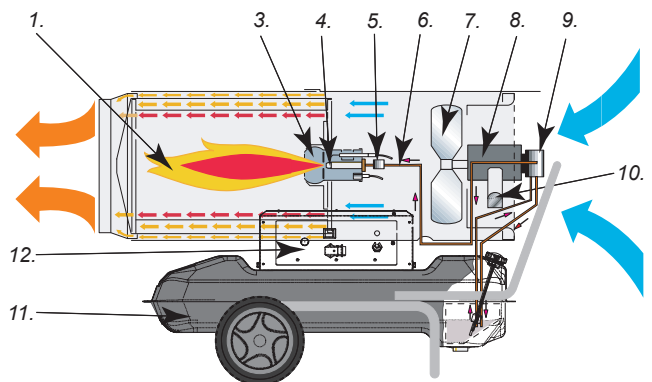
Abbildung 5 - Betriebsschema B.
